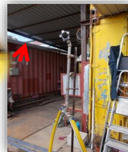
使用废弃铁枝制作固定或降尘装置
